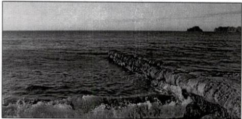
Figura 1-1. Espolón en bolsacreto construido por parte de la comunidad del sector de Playa Salguero.
